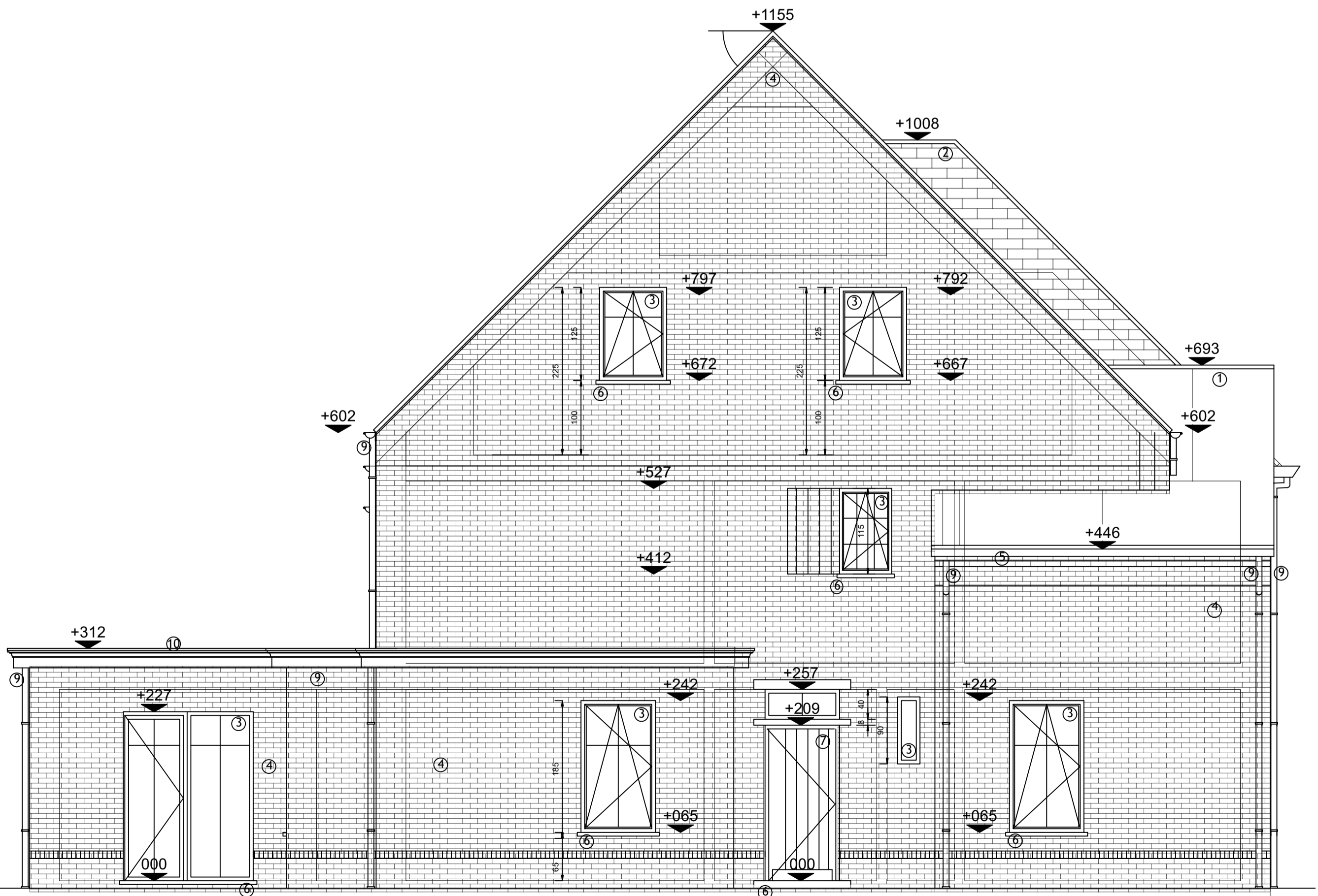
ZIJGEVEL RECHTS, LOT 3 SCHAAL 1/50
